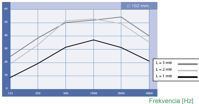
Sonoflex 102 csillapítási görbái
