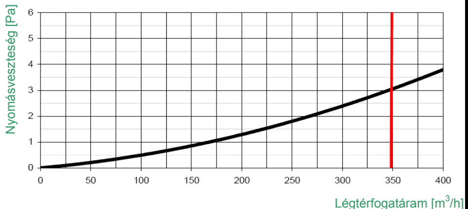
SMD 280x405 cirkulációs rács nyomásdiagramja
