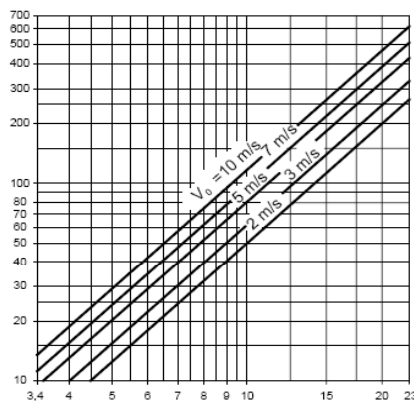
SF-05 nyomásdiagramja
