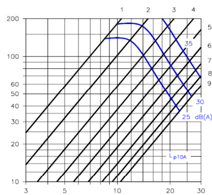
STH 100 nyomásdiagramja
