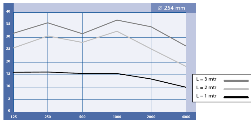
Sonoflex 254 csillapítási görbéi
