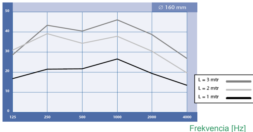
Sonoflex 160 csillapítási görbái
