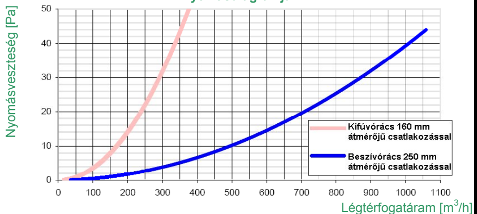
PZ 340x340 (VPF 350x350/160-nal) és PZ 340x340 (SPF 350x350/250-nel) nyomásdiagramja
