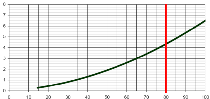
PMR 4''-10'' 250x97 padlórács nyomásdiagramja
