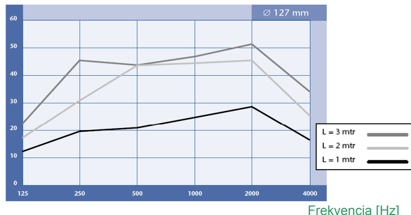
Sonoflex 127 csillapítási görbái
