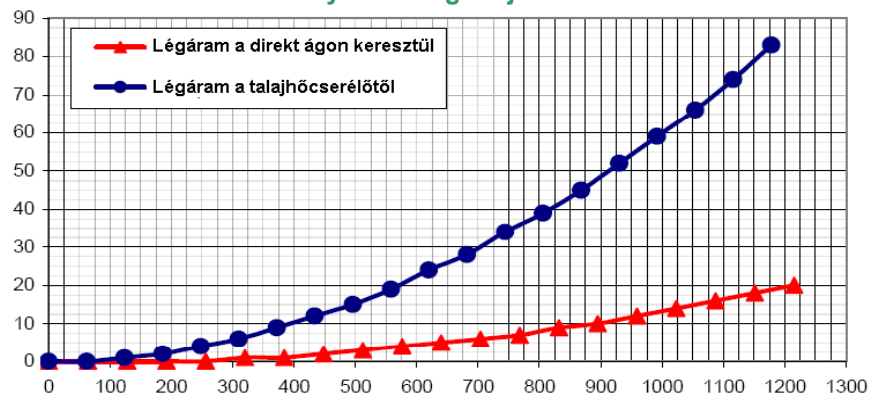
TKR 250/250/250 J, TKR 250/250/250 B, TKR 250/250/250 átellenes nyomásdiagramja
