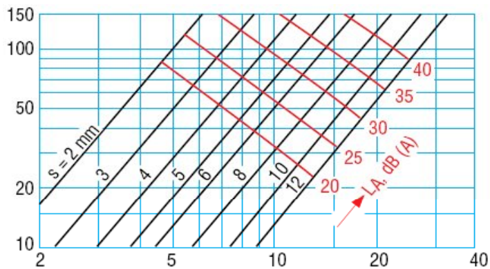
CTVK 100 nyomásdiagramja
