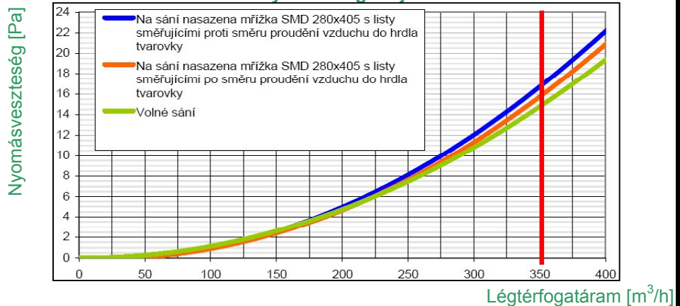
SMD 280x405 cirkulációs rács és KMI 280x405/200 beltéri dobozidom nyomásdiagramja
