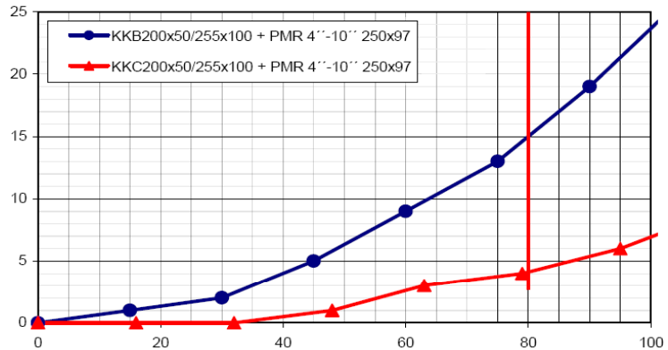
KKB és KKC dobozidomok nyomásdiagramja
