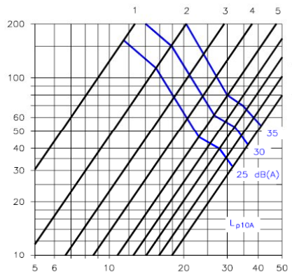
STH 125 nyomásdiagramja
