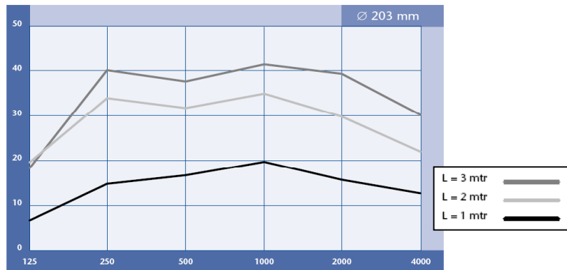
Sonoflex 203 csillapítási görbéi
